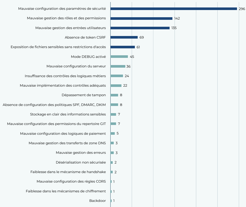
Figure 10 : Occurrences des causes des vulnérabilités
