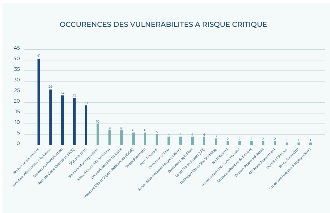
Figure 2 : Occurrences des vulnérabilités à risque critique
